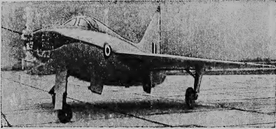
HET NIEUWE TYPE, in Engeland gebouwde, straaljager van het driehoeksvleugelmodel. Het toestel, dat lange tijd op de „geheime lijst” stond, wordt thans in het openbaar getoond. Niet bekend zijn echter de snelheid en de actie-radius.
